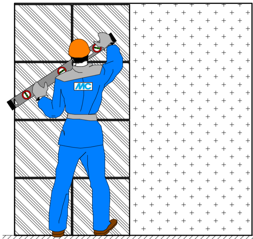
Рис.37. Последовательность работ, где: 1 – проверка ровности основания контрольной рейкой; 2, 3 – приготовление грунтовки; 4 – нанесение грунтовки на цементную штукатурку; 5 – приготовление клеевой смеси; 6, 7 – нанесение клеевой смеси на основание (захватками); 8, 9 – приклеивание керамогранитной плитки на стену (захватками); 10 – проверка облицовки при помощи уровня. ПРИМЕЧАНИЕ к рис 35.: на этапах 6-9 указано проведение работ в направлении снизу вверх, но при использовании клеев, в маркировке которых присутствует буква «Т», возможно выполнение работ в направлении сверху вниз.
