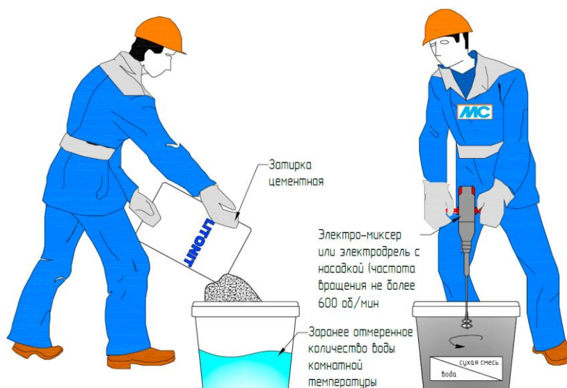
Рис. 38. Приготовление состава
