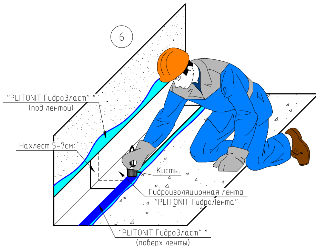
Рис.36. Последовательность работ, где: 1 - проверка ровности основания контрольной рейкой (аналогично для горизонтальной поверхности); 2 – размешивание емкости с мастикой; 3 – нанесение первого слоя мастики, разбавленной водой в пропорции 1:10, на основание; 4 – нанесение гидроизоляции на поверхность (аналогично для горизонтальной поверхности); 5 – укладка гидроизоляционной ленты на поверхность, предварительно обработанную «PLITONIT ГидроЭласт» или «PLITONIT WaterProof Standard»; 6 – поверхностная обработка ленты мастикой «PLITONIT ГидроЭласт» или «PLITONIT WaterProof Standard».
